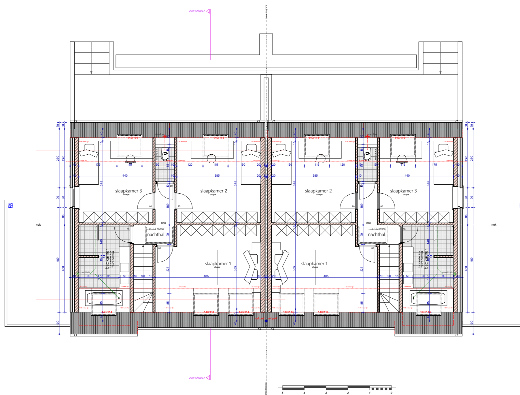
-- VERDIEPINGSPLAN nieuw -- schaal 1/100 -- A3 -- afmetingen in cm
